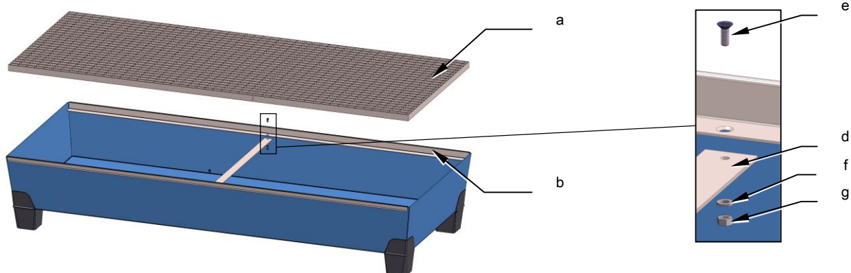
Fig. 3.3-2: Oppsamlingskar type 5
