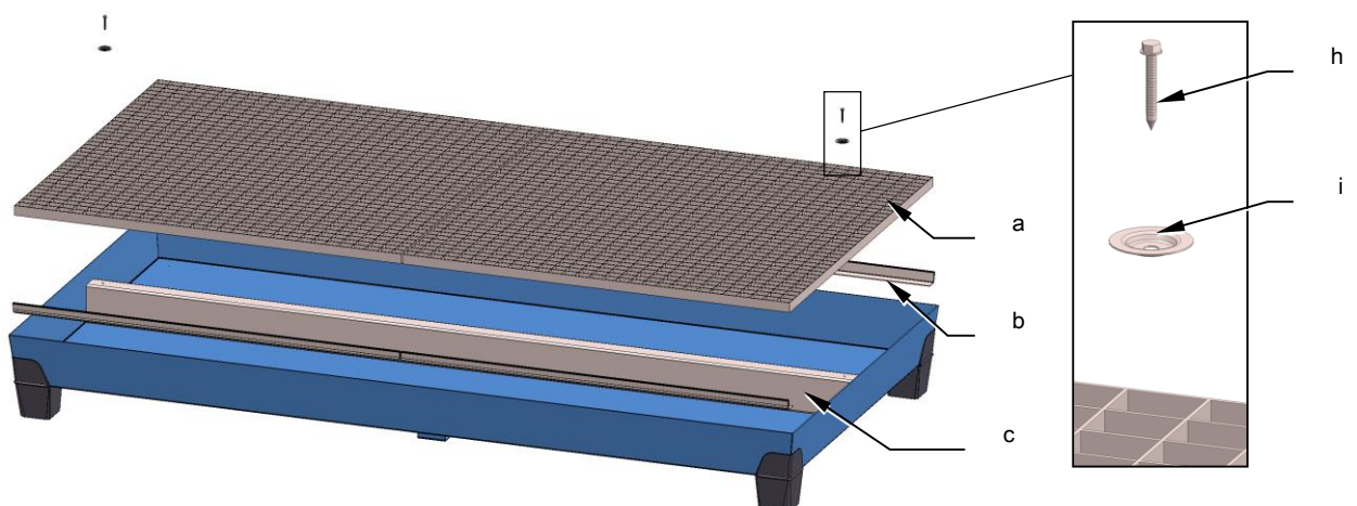
Fig. 3.3-3: cubeta de retención de tipo 7
