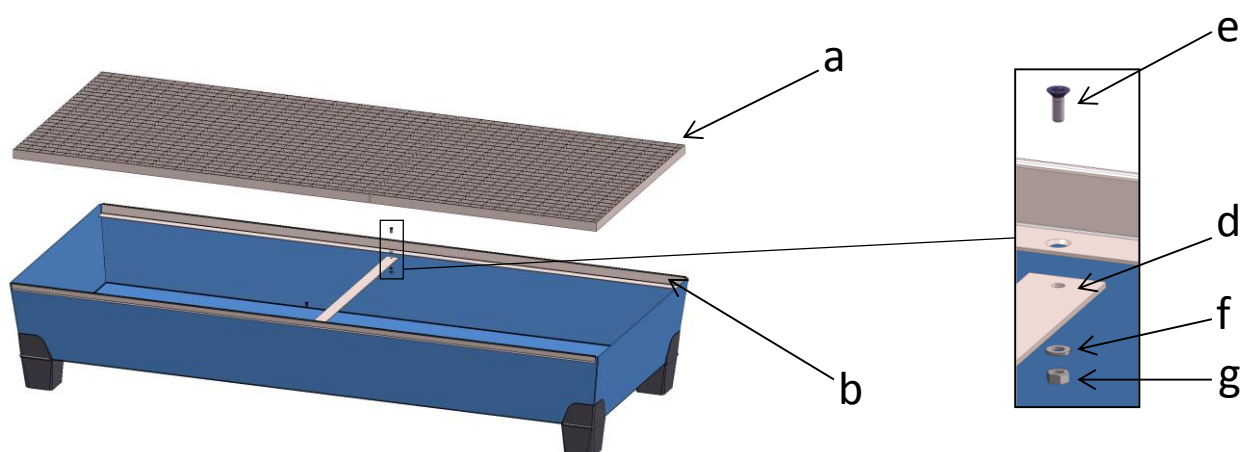
Afb. 3.3-2: opvangbak type 5
