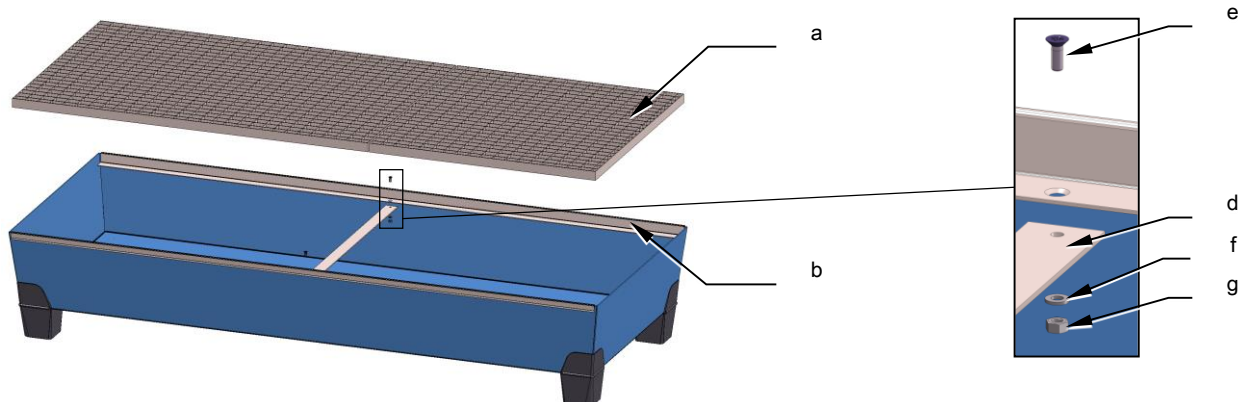
Fig. 3.3-2: Oppsamlingskar type 5
