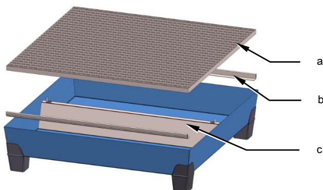
Fig. 3.3-1: Oppsamlingskar type 1, 2, 3, 4 og 6 uten pos. c
