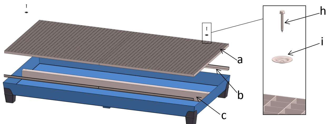
Afb. 3.3-3: opvangbak type 7
