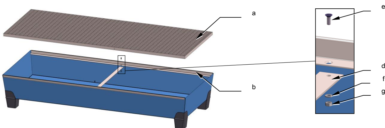
Fig. 3.3-2: Bacia de retenção Modelo 5
