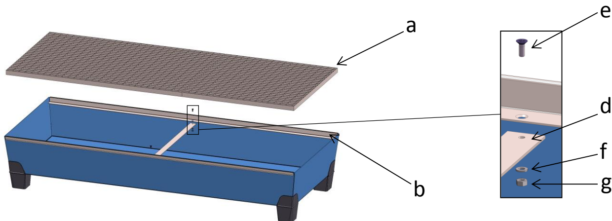
3-2. 3 ábra: 5 típusú felfogóedény
