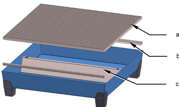
Fig. 3.3-1: Tava de colectare tip 1, 2, 3, 4 și 6 fără poz. c
