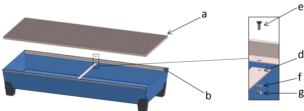
Afb. 3.3-2: opvangbak type 5
