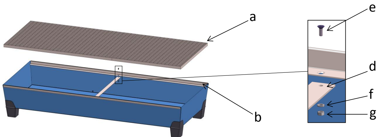
Abb. 3.3-2: Auffangwanne Typ 5
