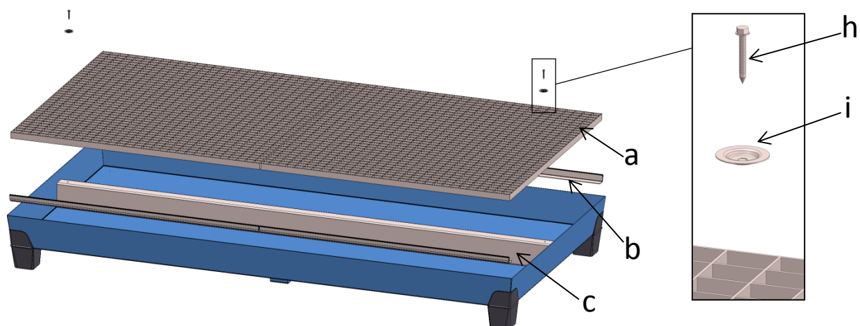
Kuva 3.3-3: Keräysallas, malli 7
