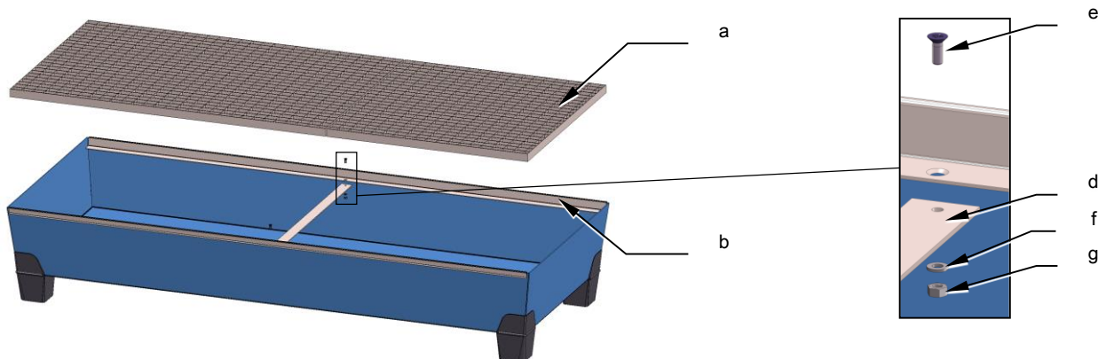
Fig. 3.3-2: Tava de colectare tip 5
