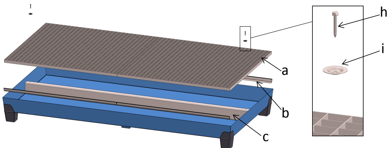
Abb. 3.3-3: Auffangwanne Typ 7
