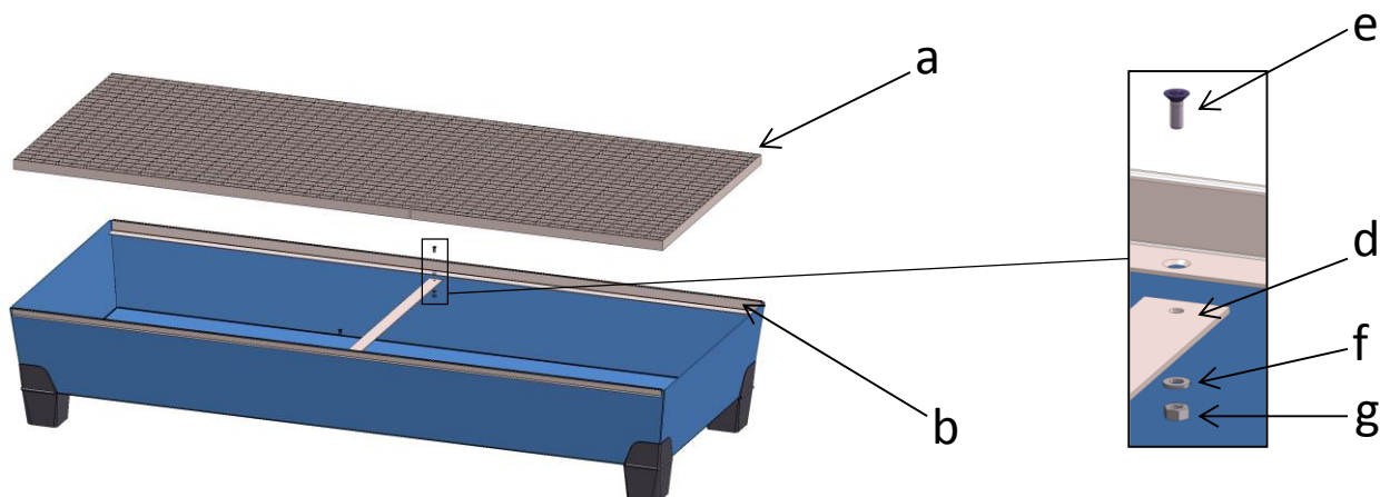
Kuva 3. 3-2: Keräysallas, malli 5
