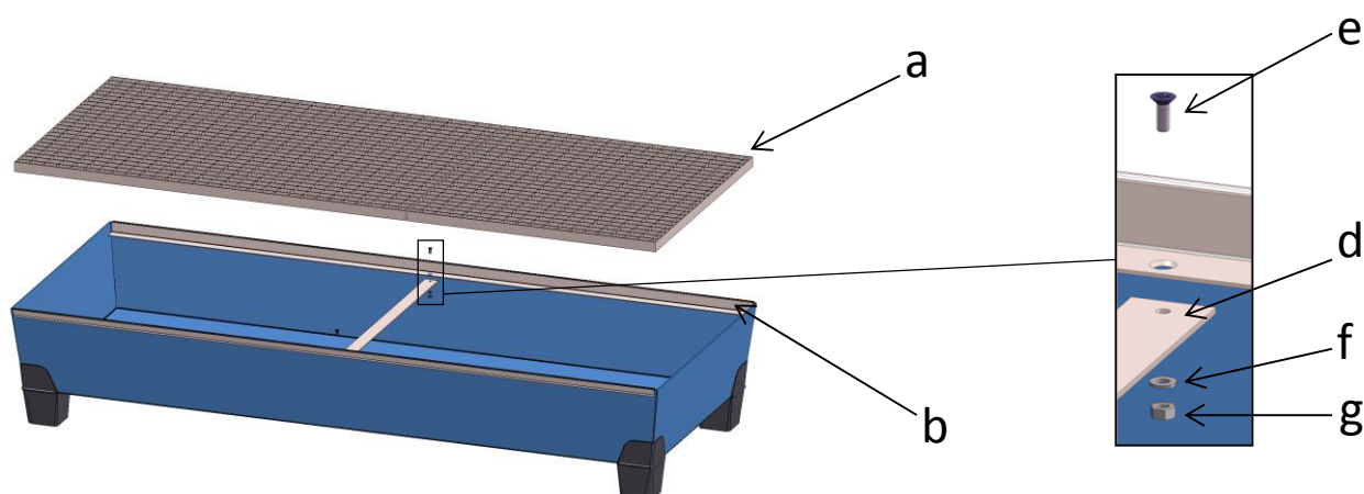
Fig. 3.3-2 : bac de rétention type 5
