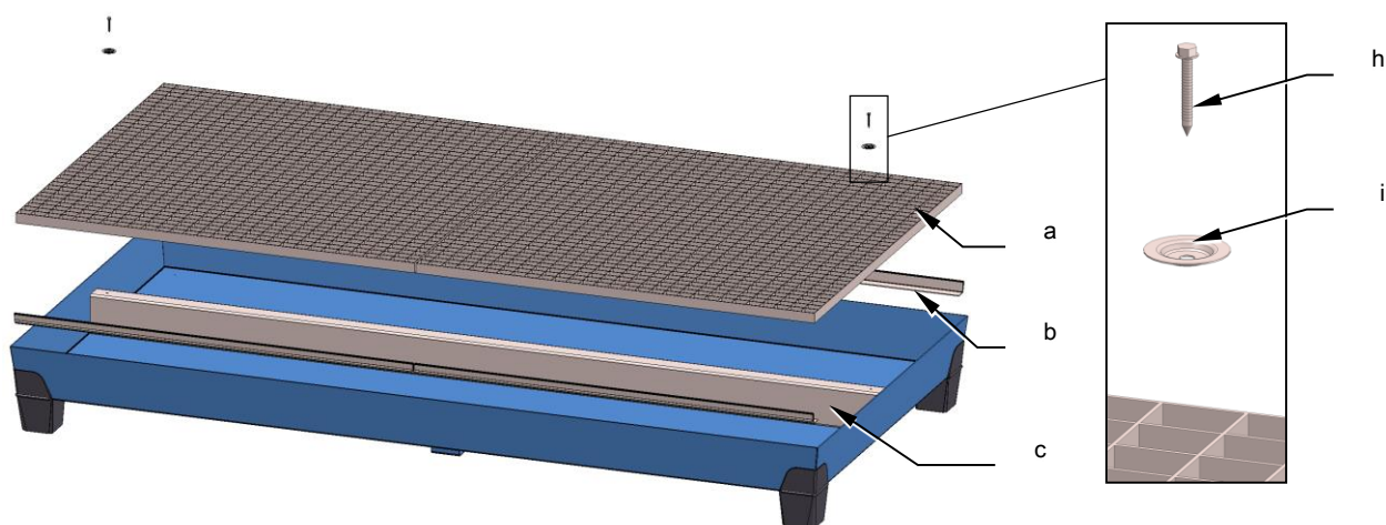
Fig. 3.3-3: Oppsamlingskar type 7
