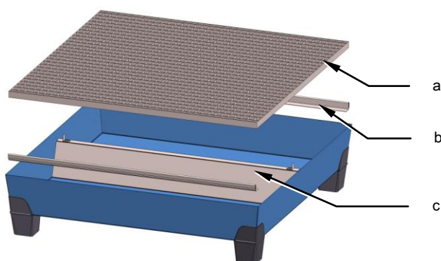
Fig. 3.3-1 : bac de rétention type 1, 2, 3, 4 et 6 sans pos. c
