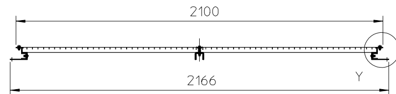
Schnitt A-A
